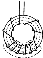
Abb. 146. Magnetische Streuung bei ungleich verteilter Wicklung.
